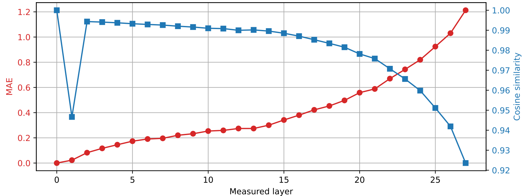
Llama-3.2-3B | Prompt 2 Spared layer 27 | Hybrid vs unquantized
