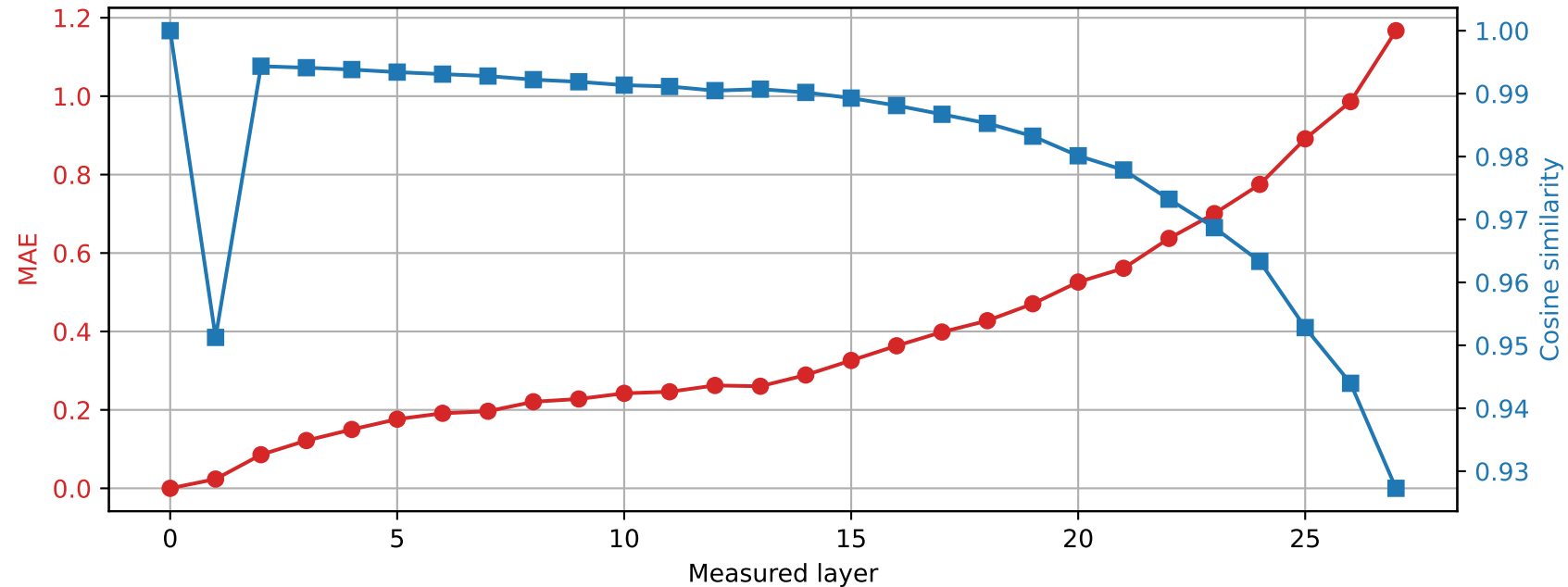
Llama-3.2-3B | Prompt 3 Spared layer 3 | Hybrid vs unquantized
