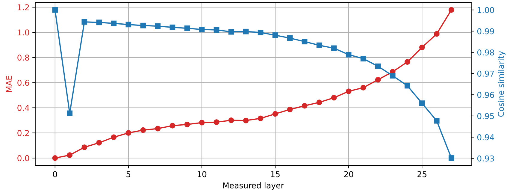
Llama-3.2-3B | Prompt 3 Spared layer 6 | Hybrid vs unquantized
