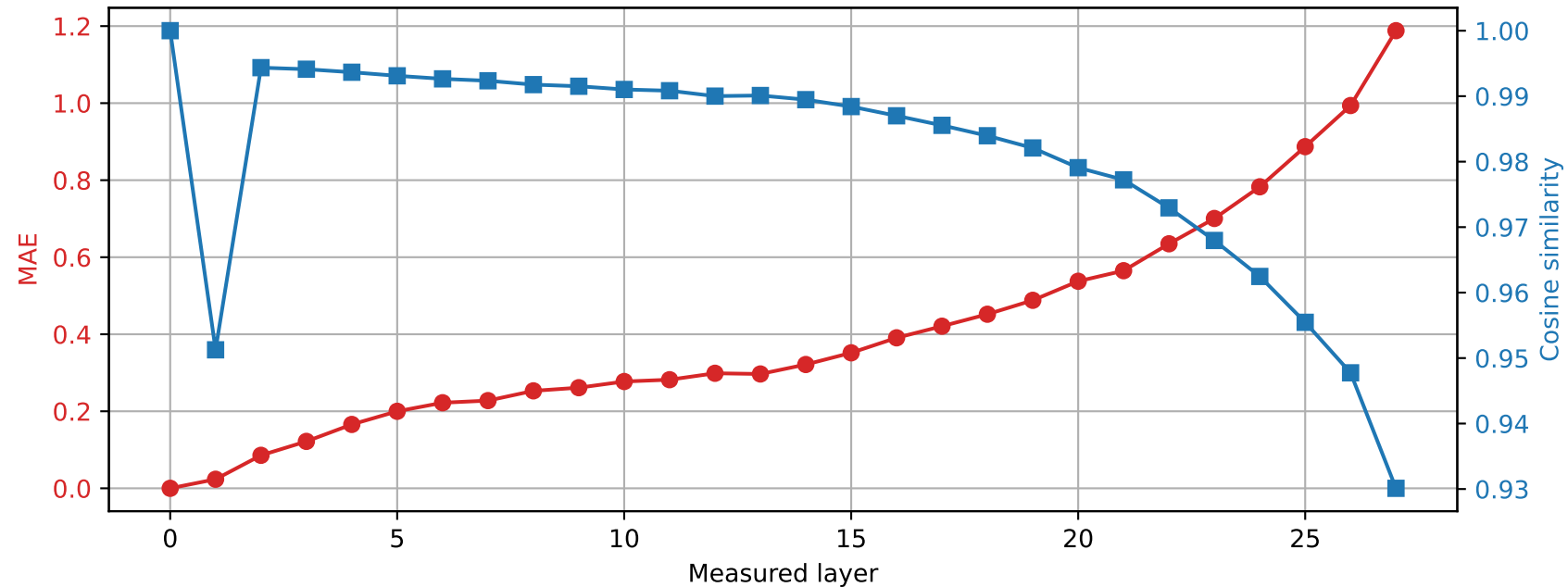
Llama-3.2-3B | Prompt 3 Spared layer 8 | Hybrid vs unquantized
