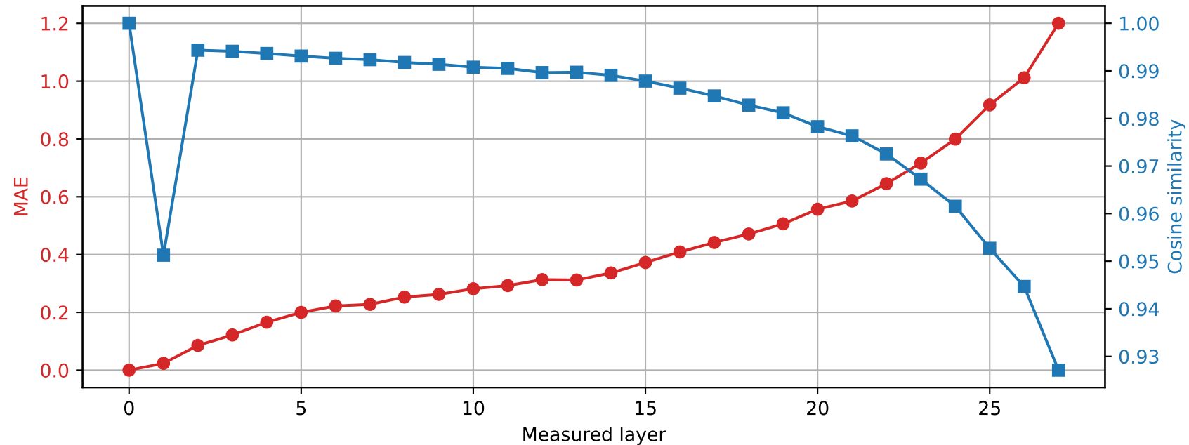
Llama-3.2-3B | Prompt 3 Spared layer 10 | Hybrid vs unquantized
