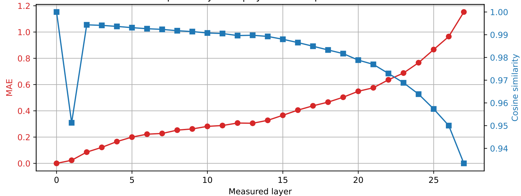
Llama-3.2-3B | Prompt 3 Spared layer 22 | Hybrid vs unquantized
