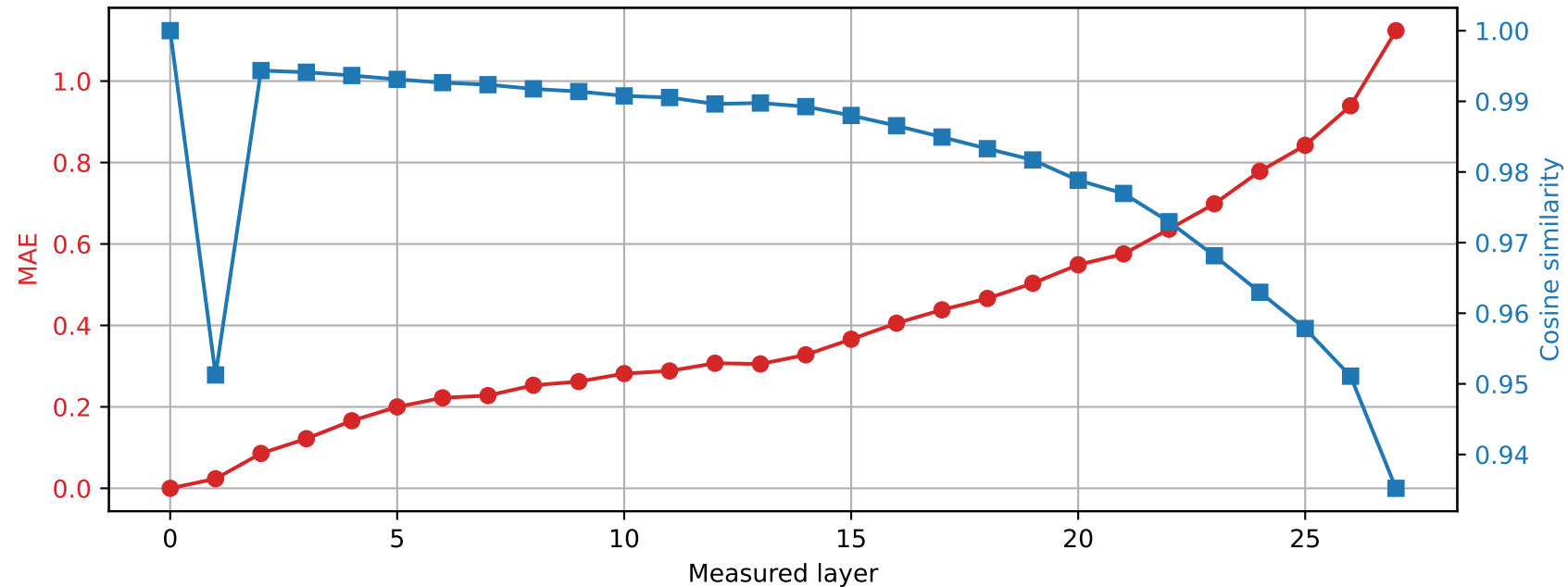
Llama-3.2-3B | Prompt 3 Spared layer 24 | Hybrid vs unquantized
