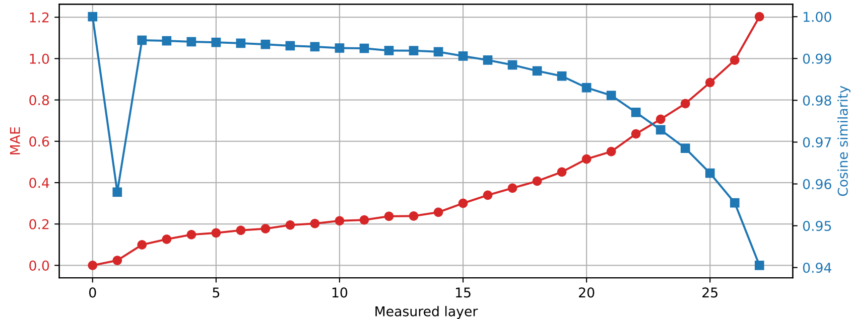
Llama-3.2-3B | Prompt 4 Spared layer 4 | Hybrid vs unquantized
