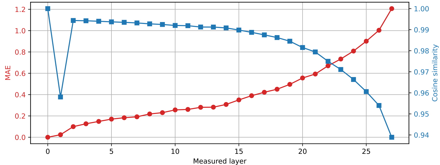
Llama-3.2-3B | Prompt 4 Spared layer 14 | Hybrid vs unquantized
