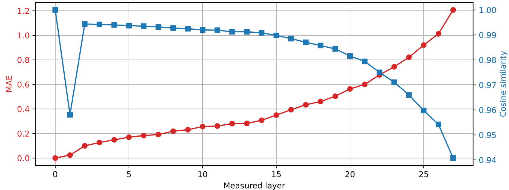
Llama-3.2-3B | Prompt 4 Spared layer 16 | Hybrid vs unquantized
