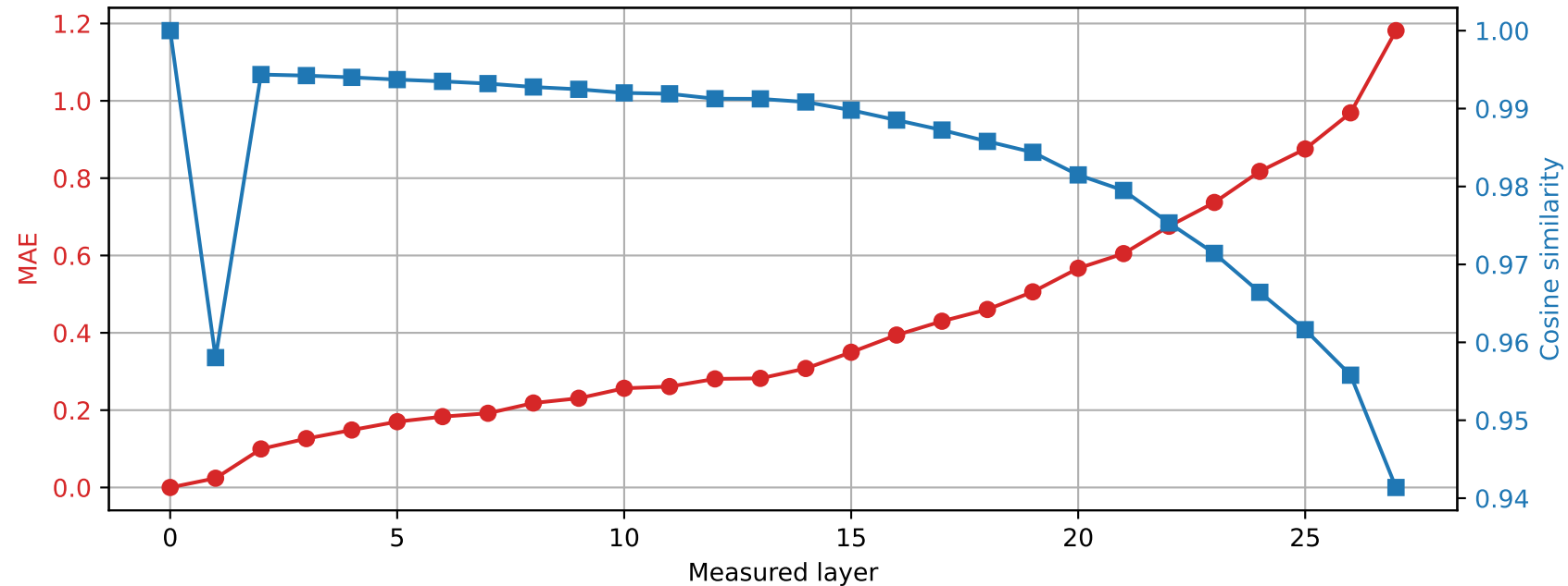
Llama-3.2-3B | Prompt 4 Spared layer 24 | Hybrid vs unquantized
