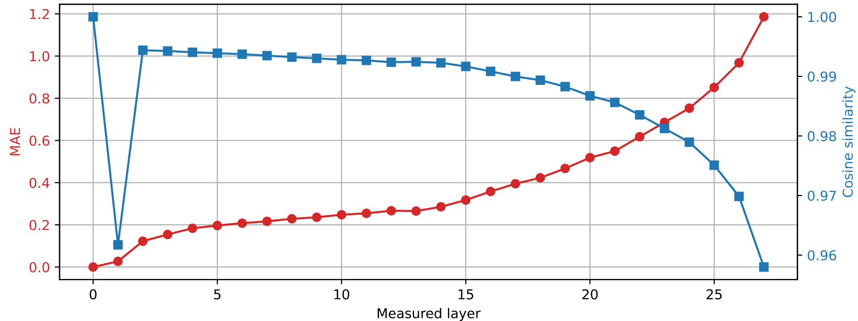
Llama-3.2-3B | Prompt 0 Spared layer 4 | Hybrid vs unquantized
