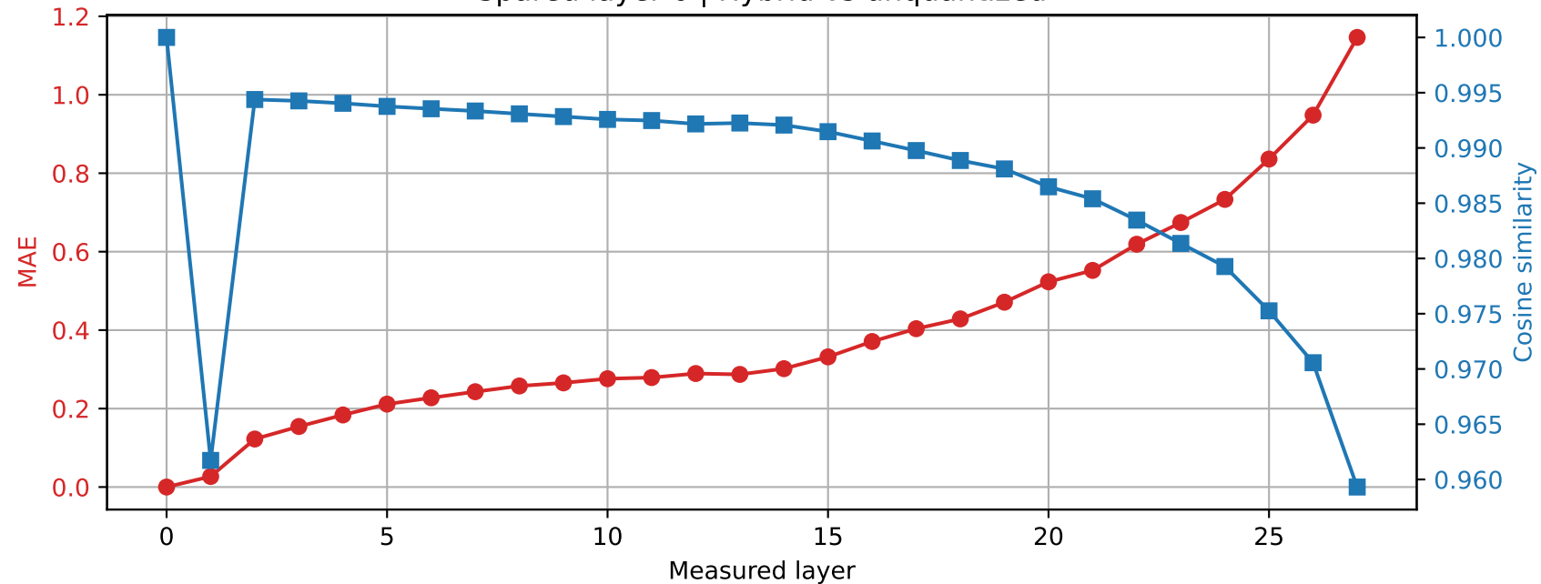
Llama-3.2-3B | Prompt 0 Spared layer 6 | Hybrid vs unquantized
