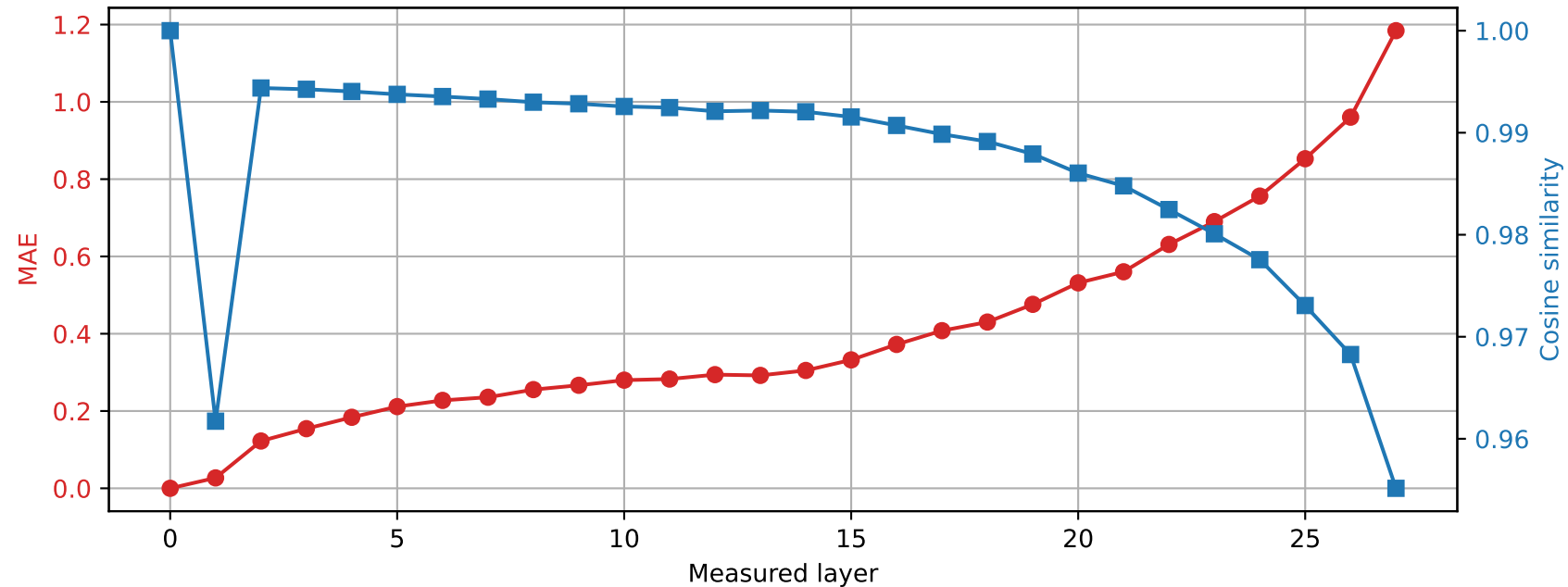
Llama-3.2-3B | Prompt 0 Spared layer 8 | Hybrid vs unquantized
