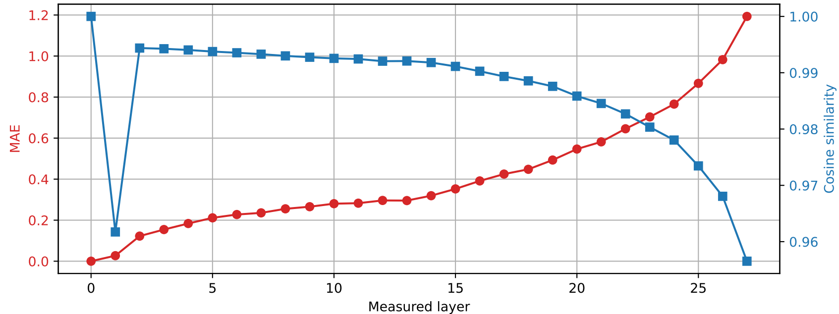
Llama-3.2-3B | Prompt 0 Spared layer 9 | Hybrid vs unquantized
