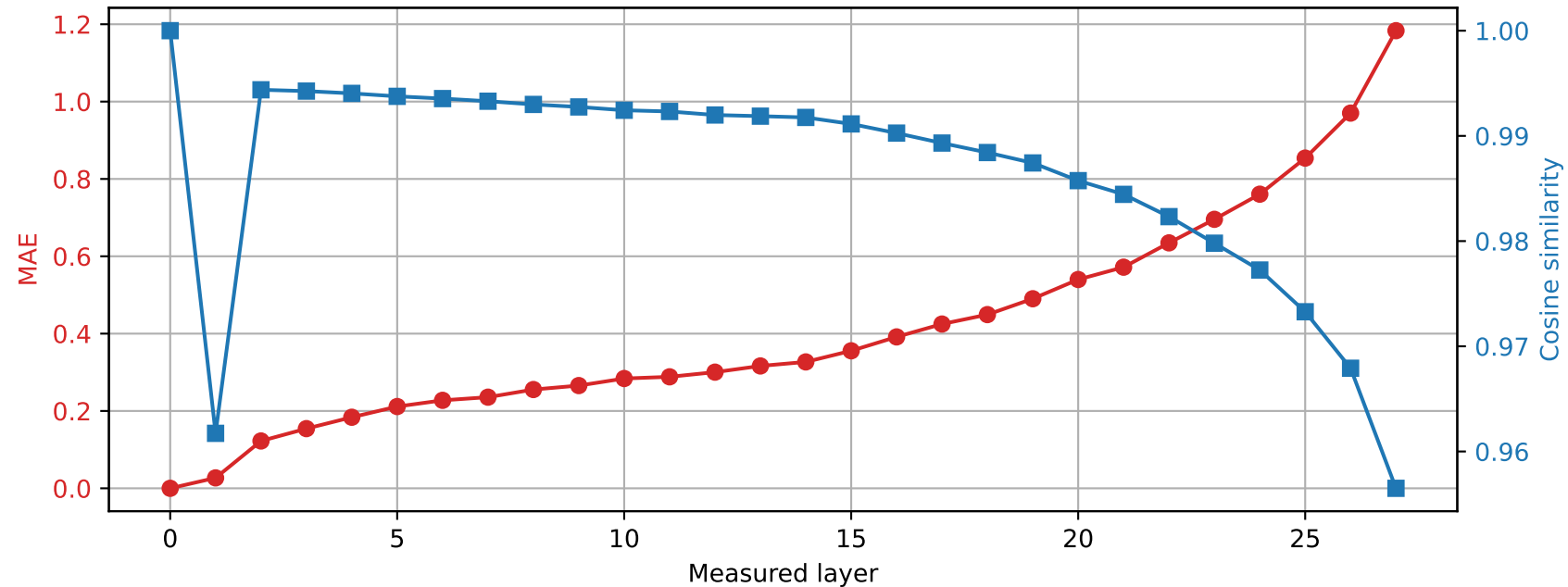
Llama-3.2-3B | Prompt 0 Spared layer 12 | Hybrid vs unquantized
