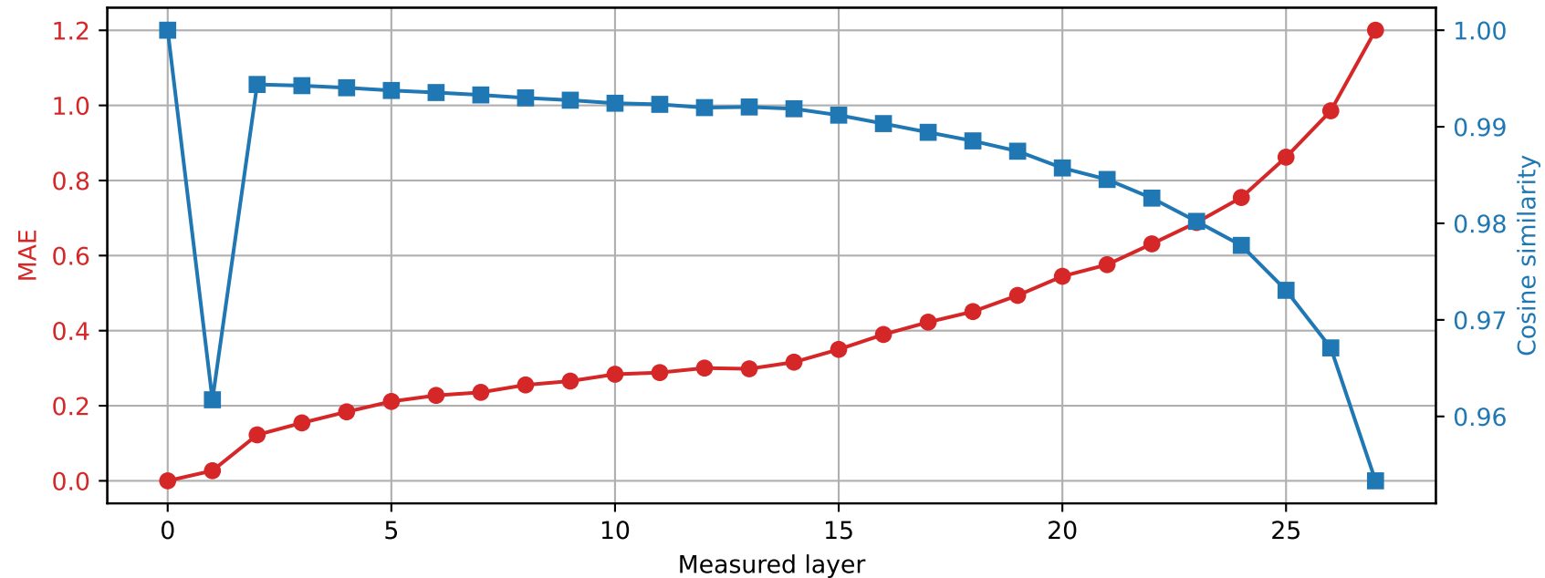
Llama-3.2-3B | Prompt 0 Spared layer 26 | Hybrid vs unquantized
