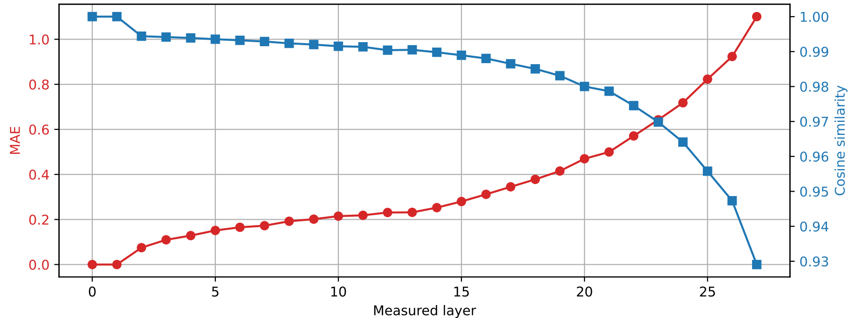
Llama-3.2-3B | Prompt 1 Spared layer 0 | Hybrid vs unquantized
