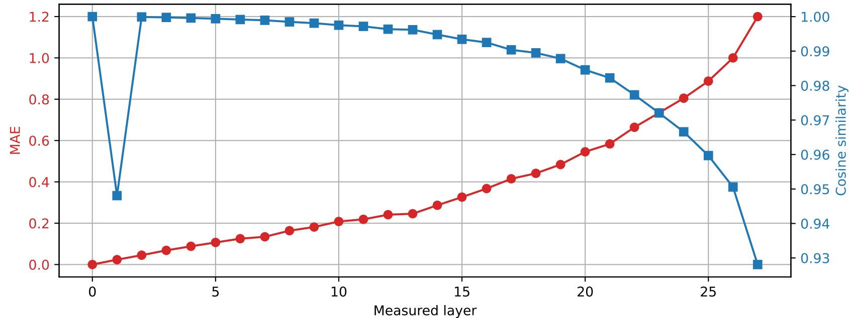
Llama-3.2-3B | Prompt 1 Spared layer 1 | Hybrid vs unquantized
