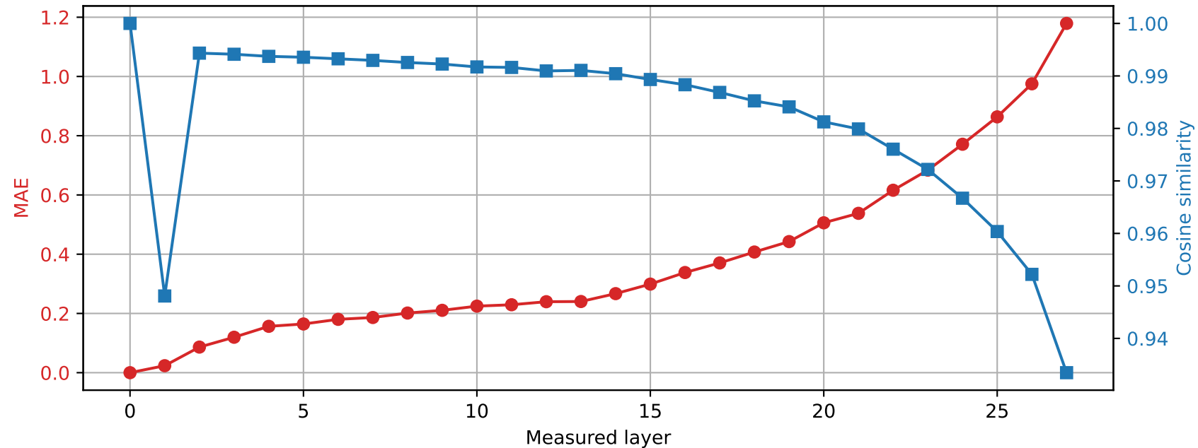
Llama-3.2-3B | Prompt 1 Spared layer 4 | Hybrid vs unquantized
