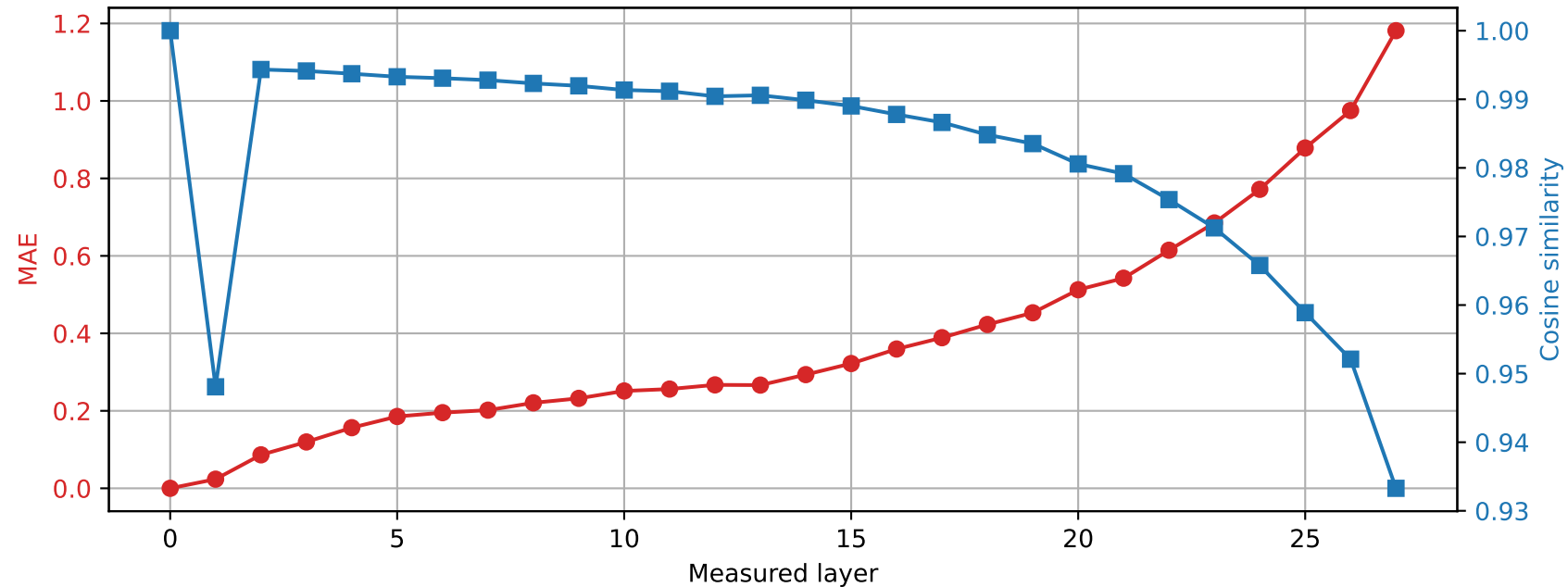
Llama-3.2-3B | Prompt 1 Spared layer 5 | Hybrid vs unquantized
