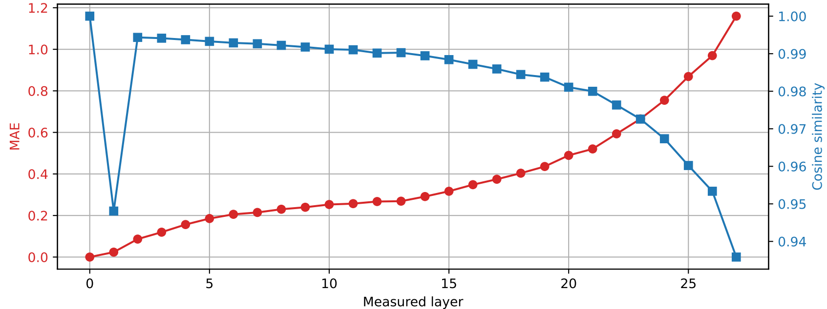
Llama-3.2-3B | Prompt 1 Spared layer 6 | Hybrid vs unquantized
