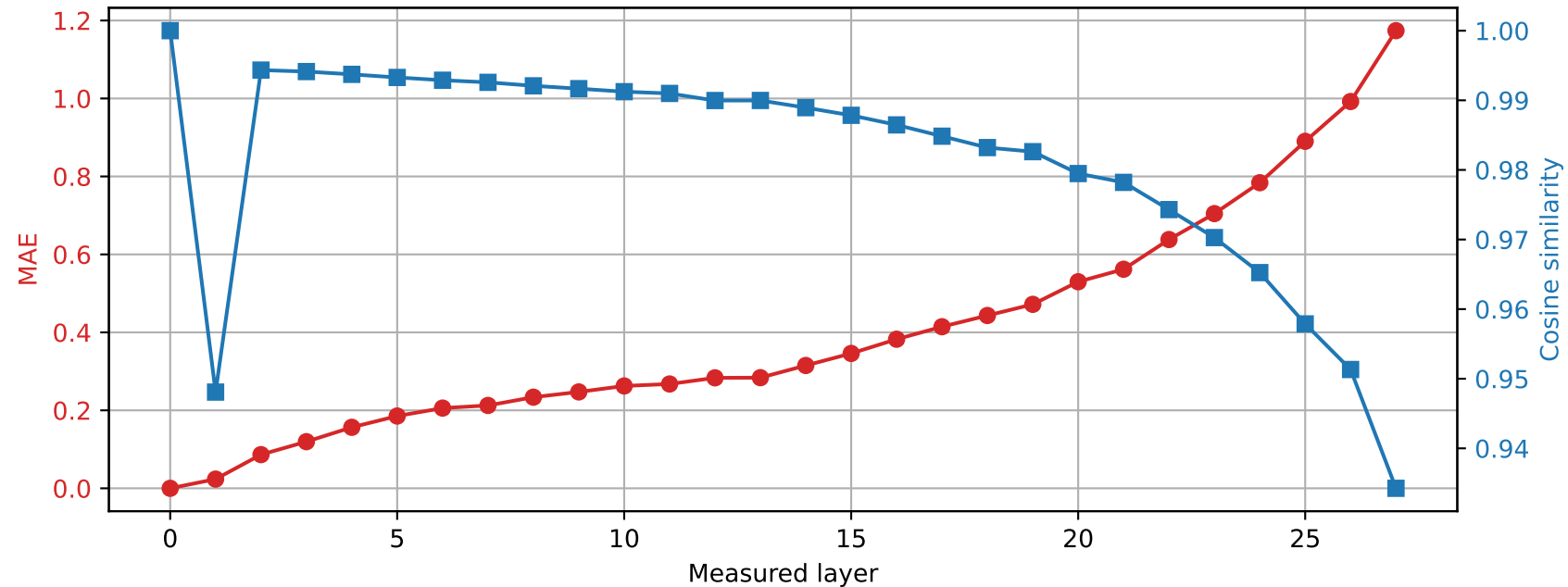
Llama-3.2-3B | Prompt 1 Spared layer 9 | Hybrid vs unquantized
