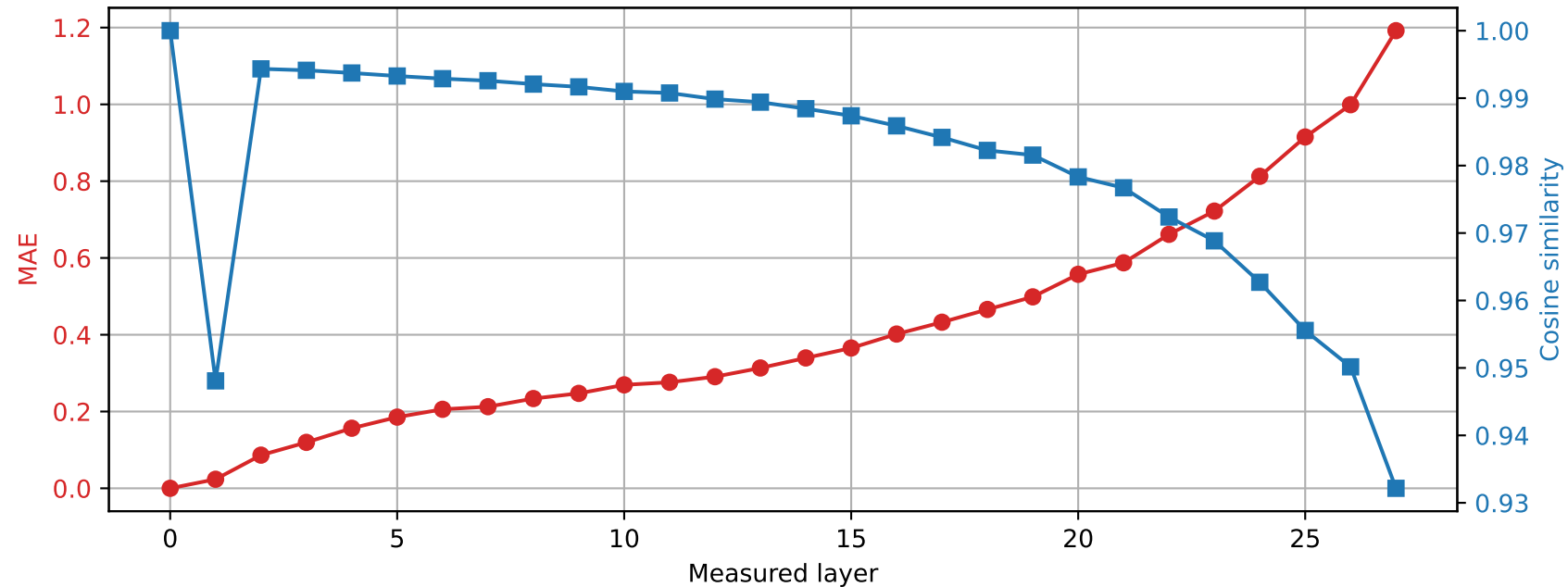
Llama-3.2-3B | Prompt 1 Spared layer 12 | Hybrid vs unquantized
