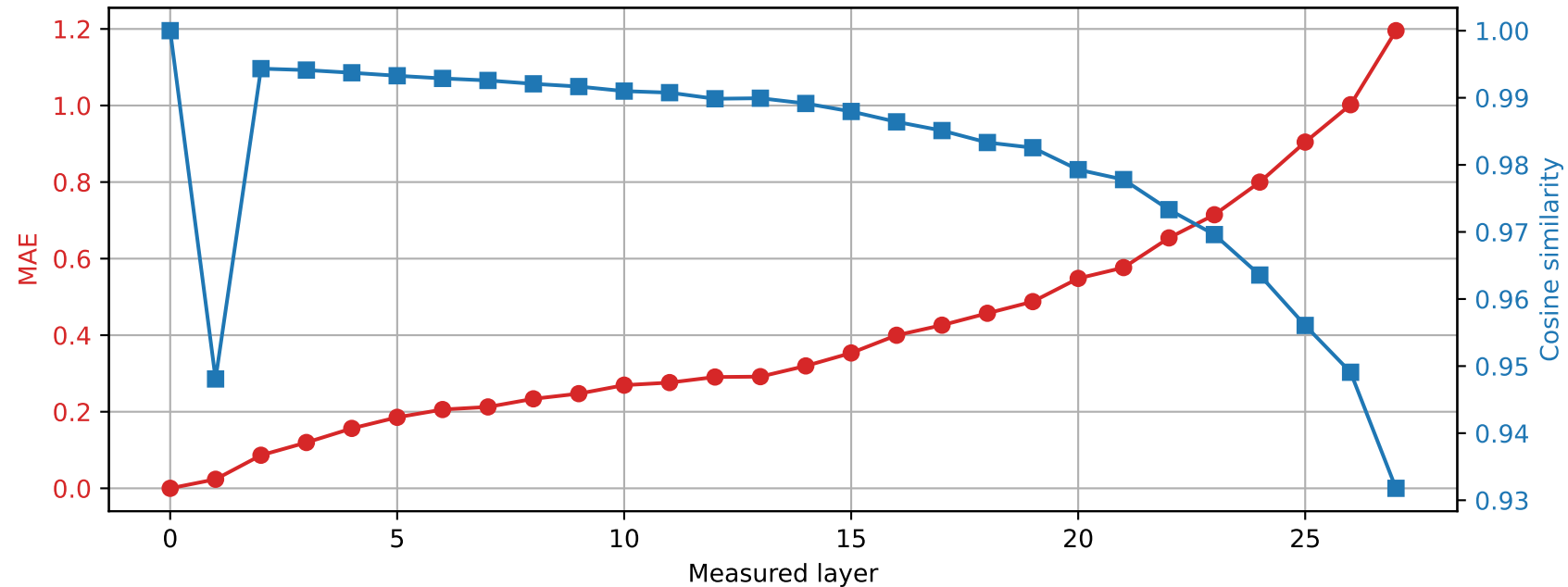
Llama-3.2-3B | Prompt 1 Spared layer 15 | Hybrid vs unquantized
