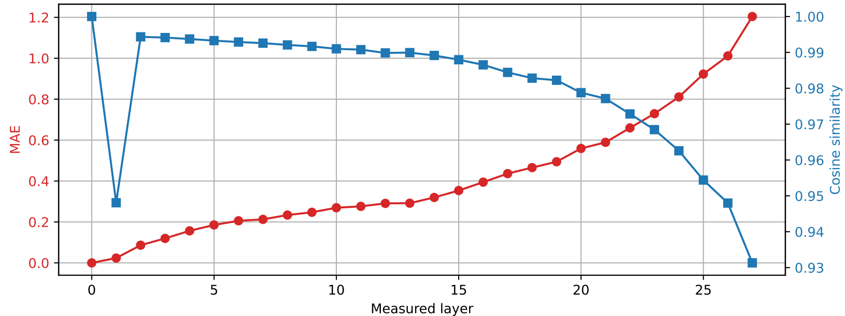
Llama-3.2-3B | Prompt 1 Spared layer 16 | Hybrid vs unquantized
