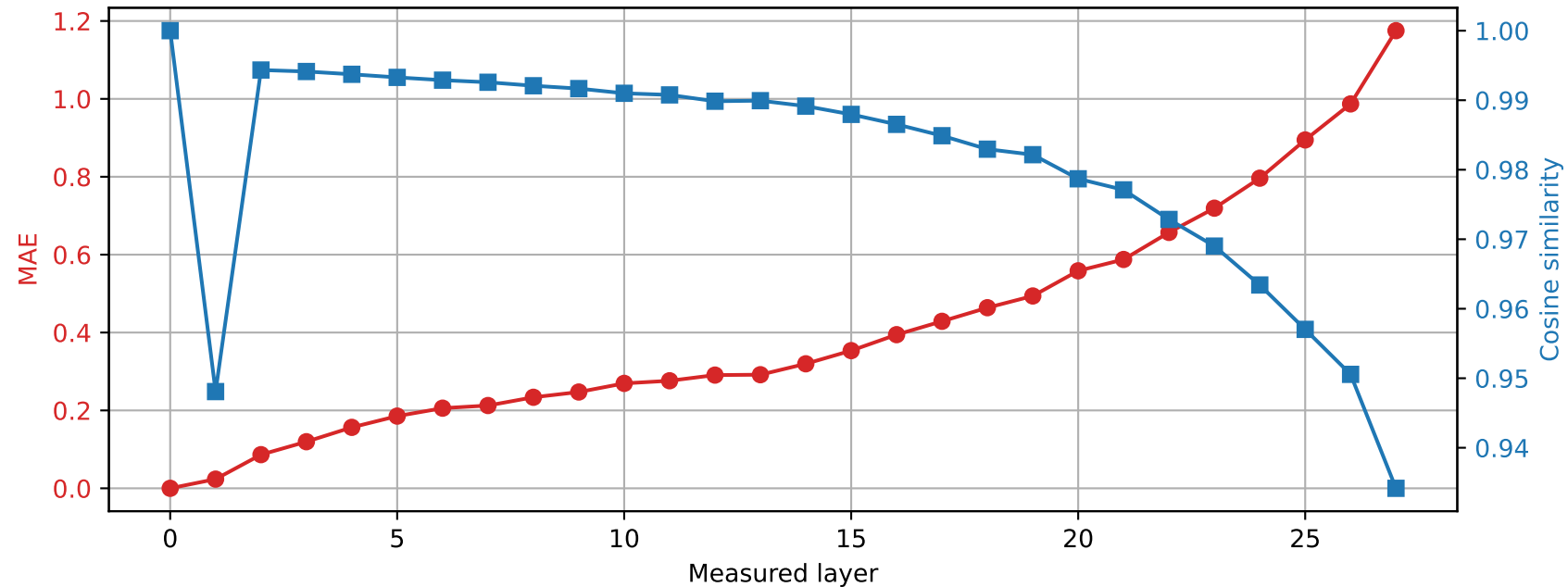
Llama-3.2-3B | Prompt 1 Spared layer 19 | Hybrid vs unquantized
