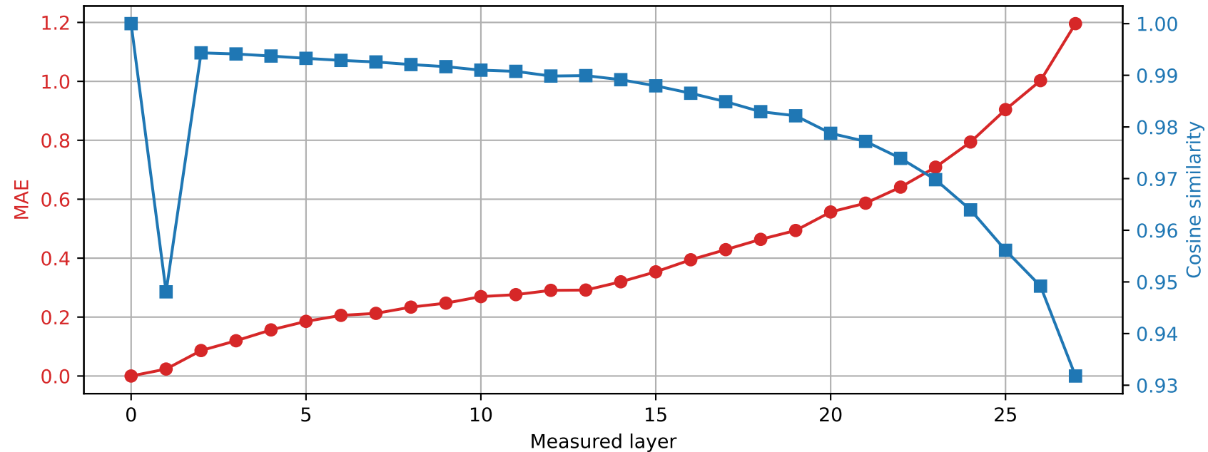
Llama-3.2-3B | Prompt 1 Spared layer 21 | Hybrid vs unquantized
