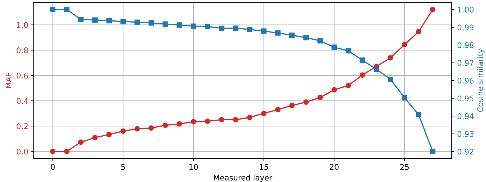
Llama-3.2-3B | Prompt 2 Spared layer 0 | Hybrid vs unquantized
