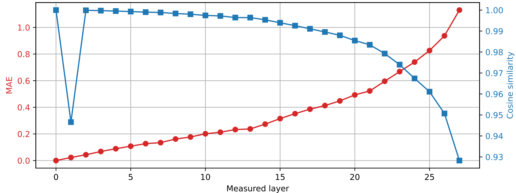
Llama-3.2-3B | Prompt 2 Spared layer 1 | Hybrid vs unquantized
