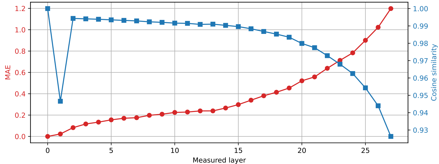
Llama-3.2-3B | Prompt 2 Spared layer 3 | Hybrid vs unquantized
