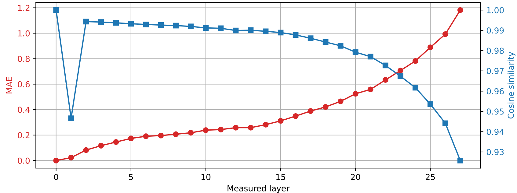
Llama-3.2-3B | Prompt 2 Spared layer 7 | Hybrid vs unquantized
