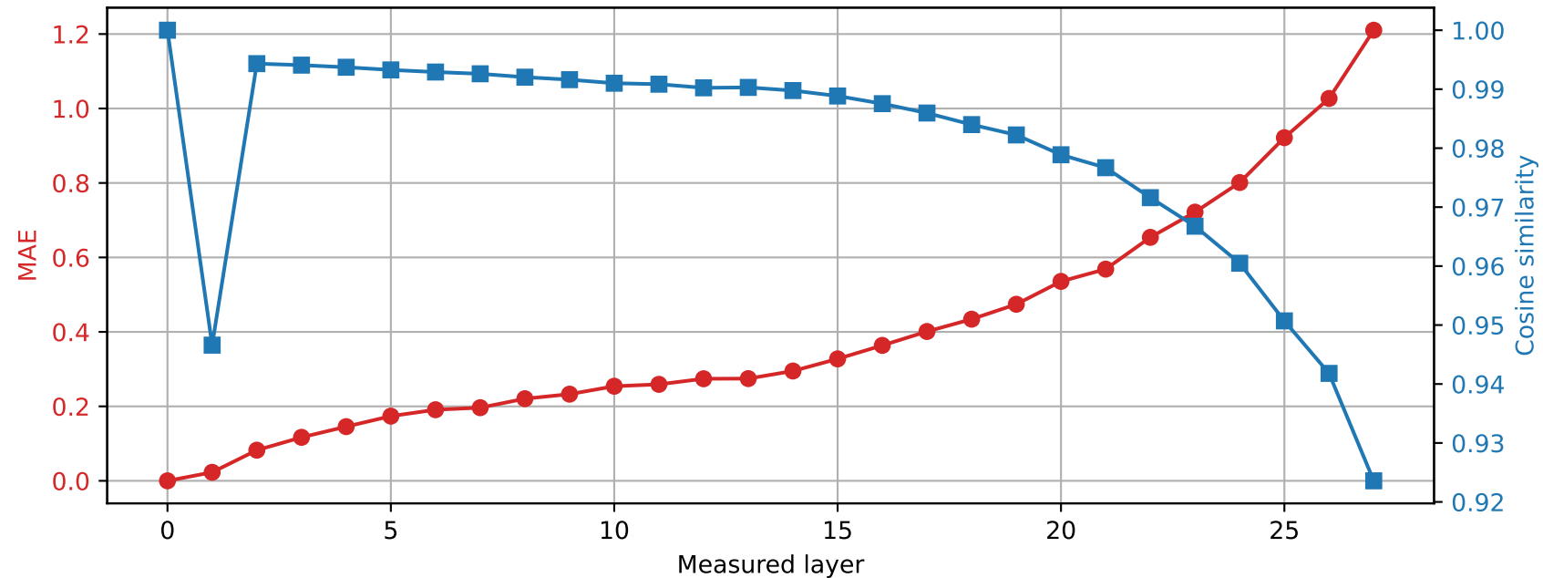
Llama-3.2-3B | Prompt 2 Spared layer 11 | Hybrid vs unquantized
