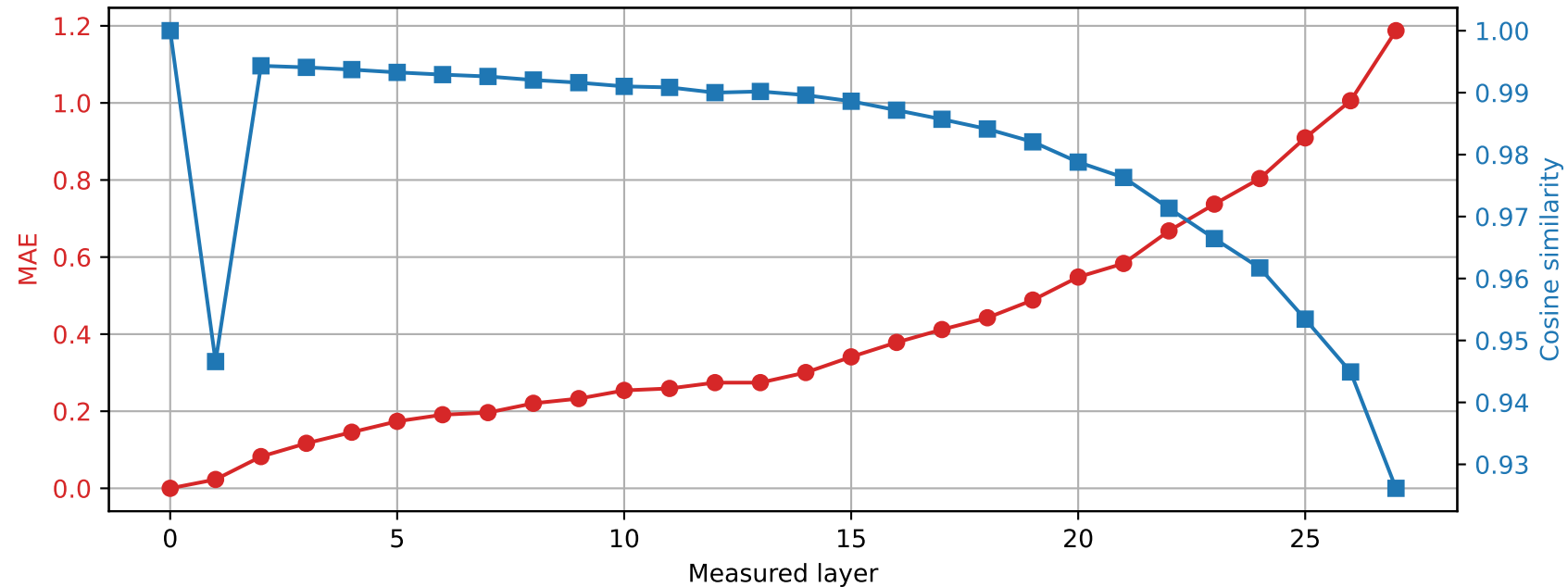
Llama-3.2-3B | Prompt 2 Spared layer 14 | Hybrid vs unquantized
