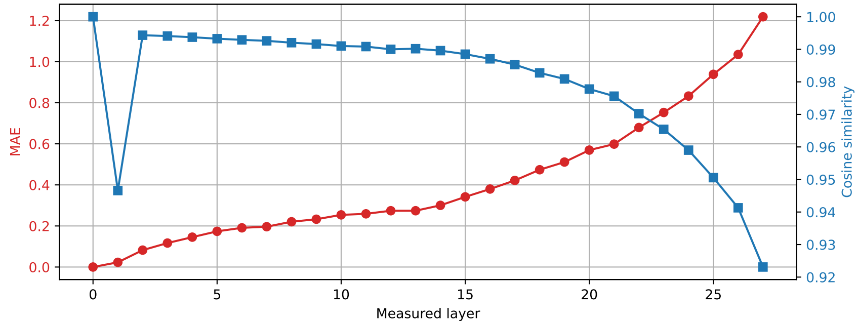
Llama-3.2-3B | Prompt 2 Spared layer 17 | Hybrid vs unquantized
