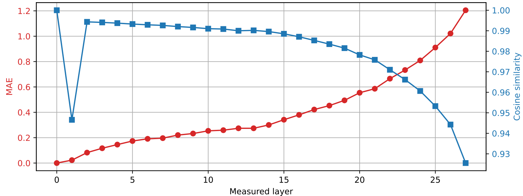
Llama-3.2-3B | Prompt 2 Spared layer 18 | Hybrid vs unquantized
