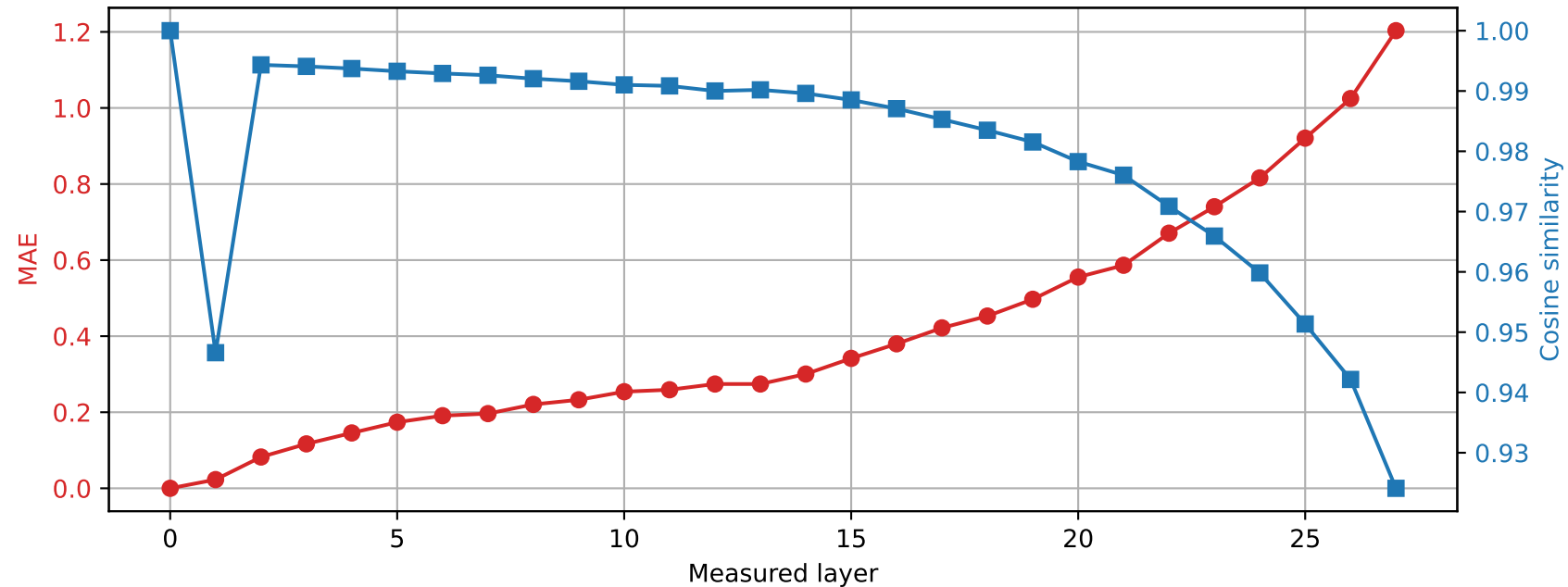
Llama-3.2-3B | Prompt 2 Spared layer 19 | Hybrid vs unquantized
