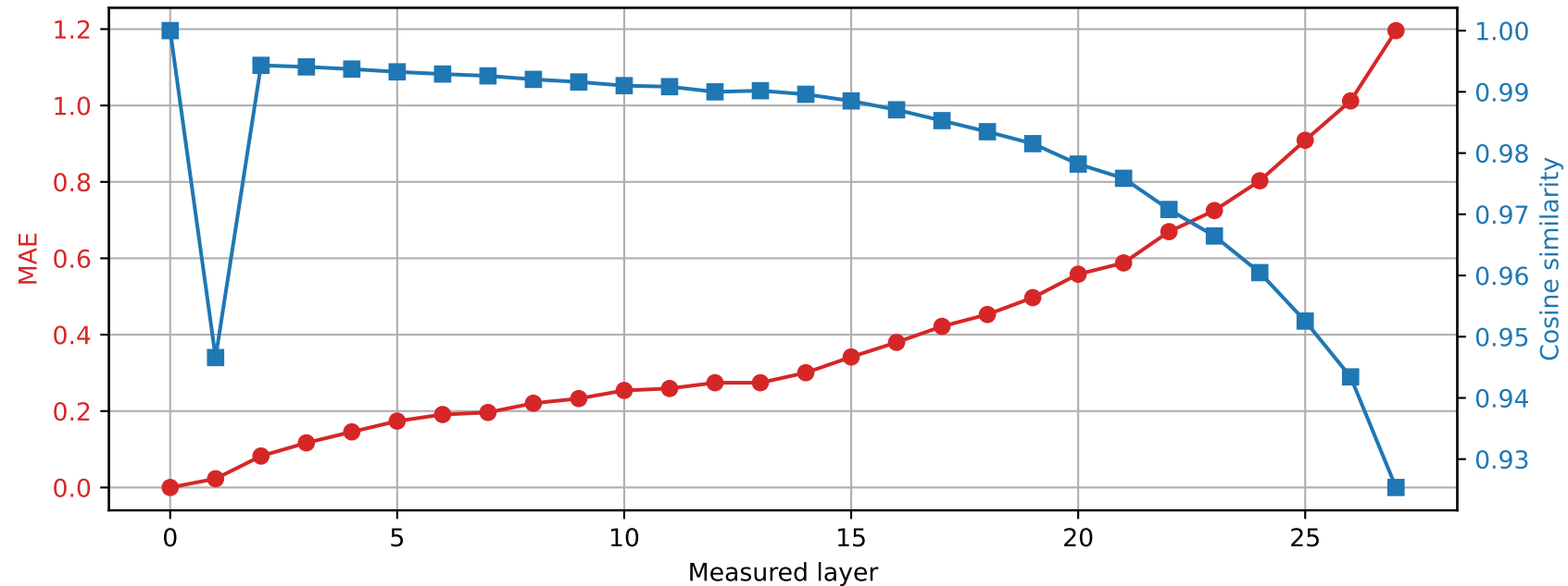
Llama-3.2-3B | Prompt 2 Spared layer 22 | Hybrid vs unquantized
