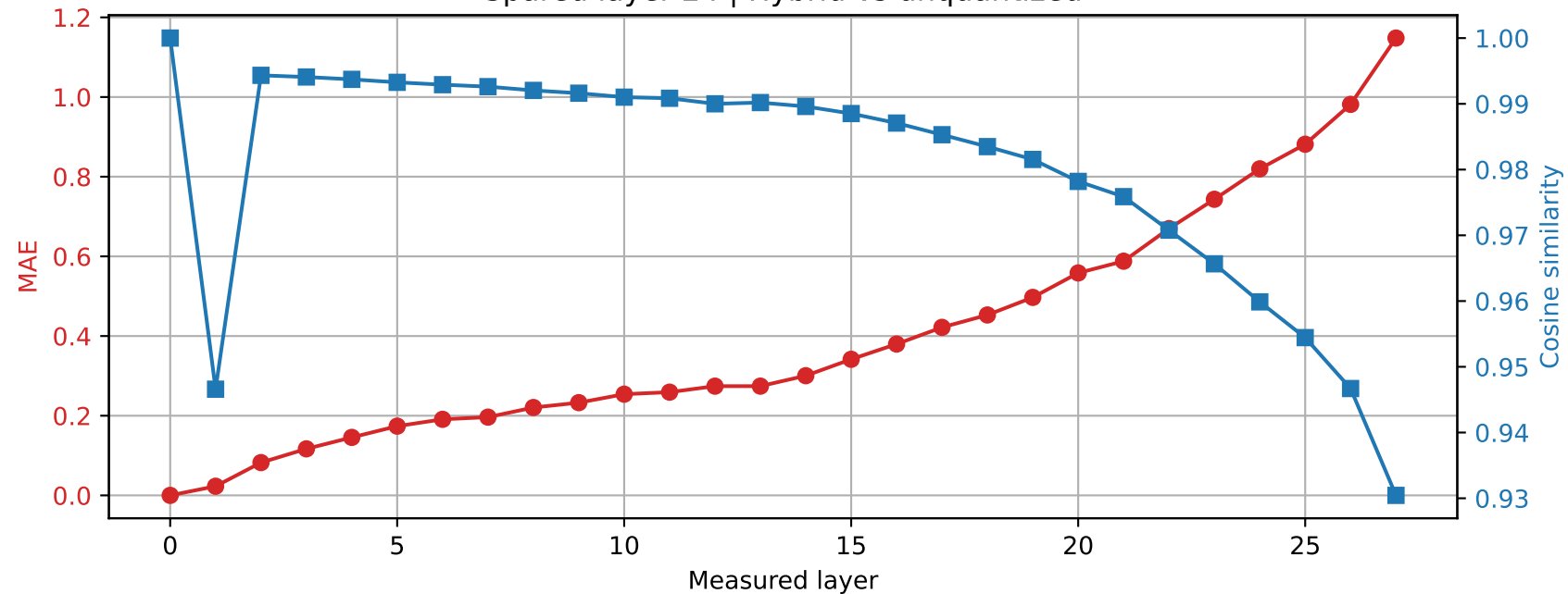
Llama-3.2-3B | Prompt 2 Spared layer 24 | Hybrid vs unquantized
