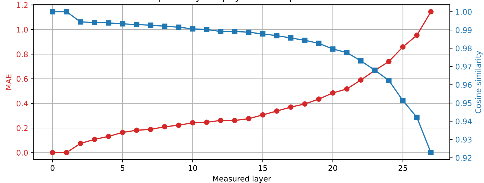
Llama-3.2-3B | Prompt 3 Spared layer 0 | Hybrid vs unquantized
