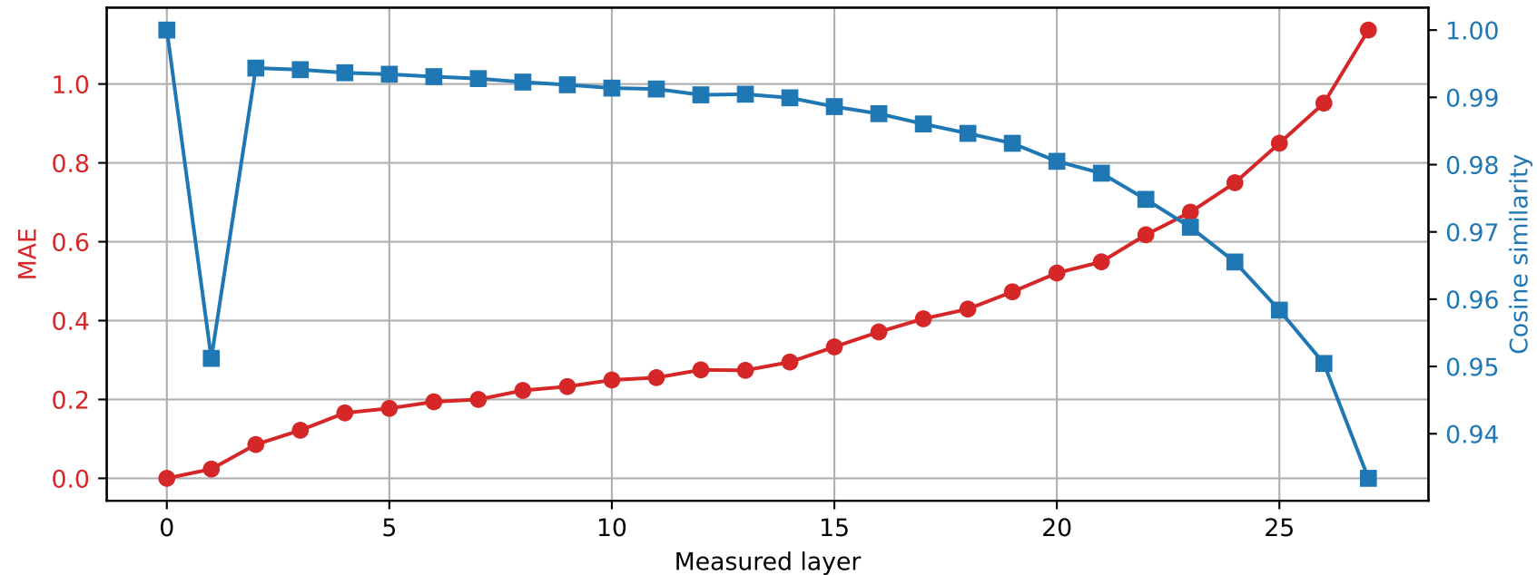
Llama-3.2-3B | Prompt 3 Spared layer 4 | Hybrid vs unquantized
