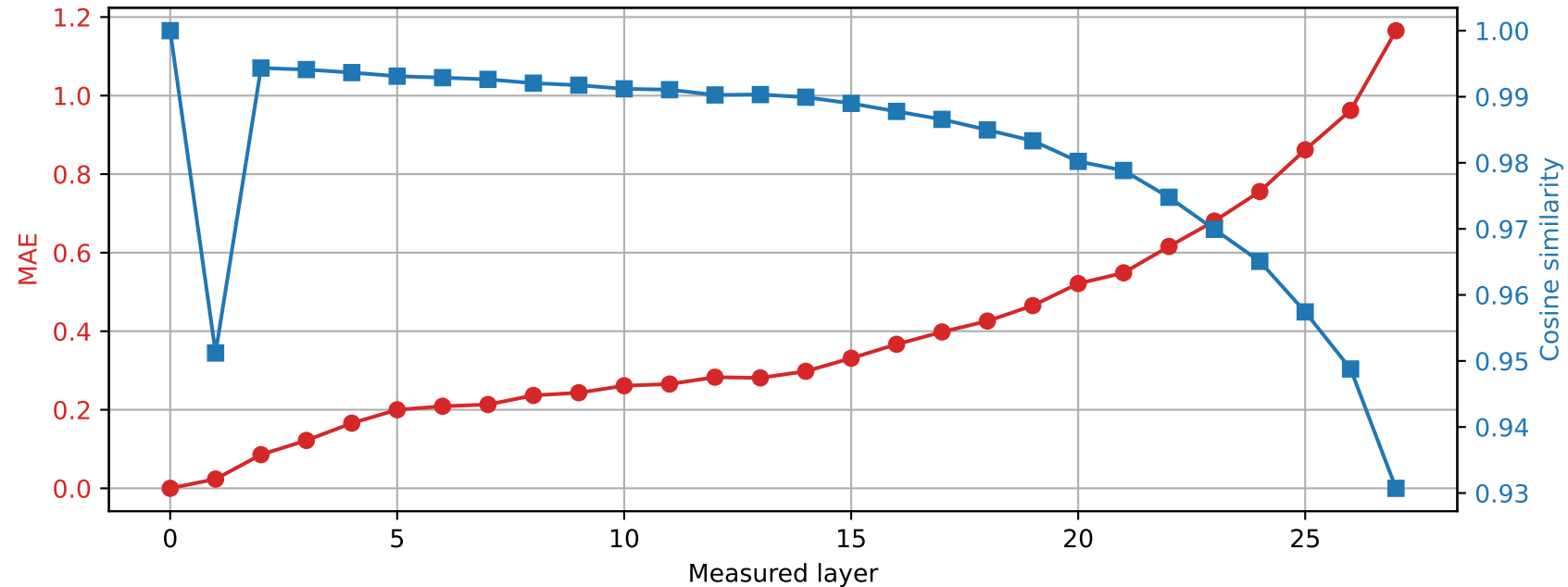
Llama-3.2-3B | Prompt 3 Spared layer 5 | Hybrid vs unquantized
