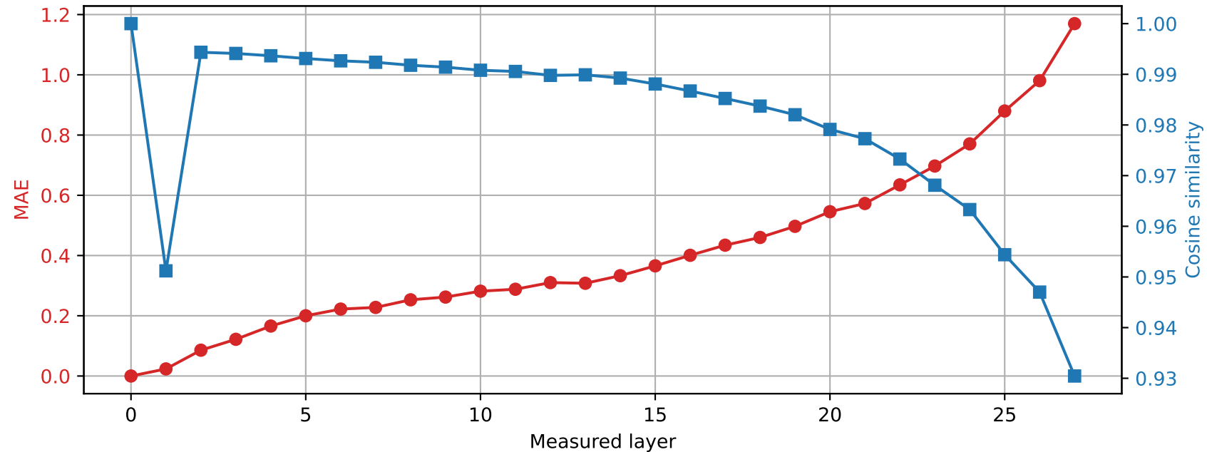
Llama-3.2-3B | Prompt 3 Spared layer 11 | Hybrid vs unquantized
