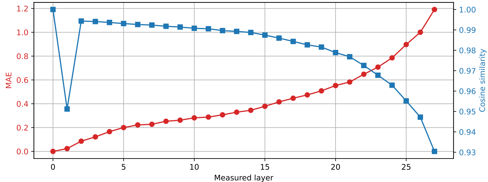
Llama-3.2-3B | Prompt 3 Spared layer 12 | Hybrid vs unquantized
