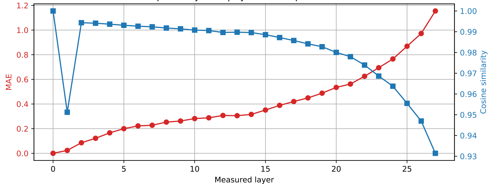
Llama-3.2-3B | Prompt 3 Spared layer 13 | Hybrid vs unquantized
