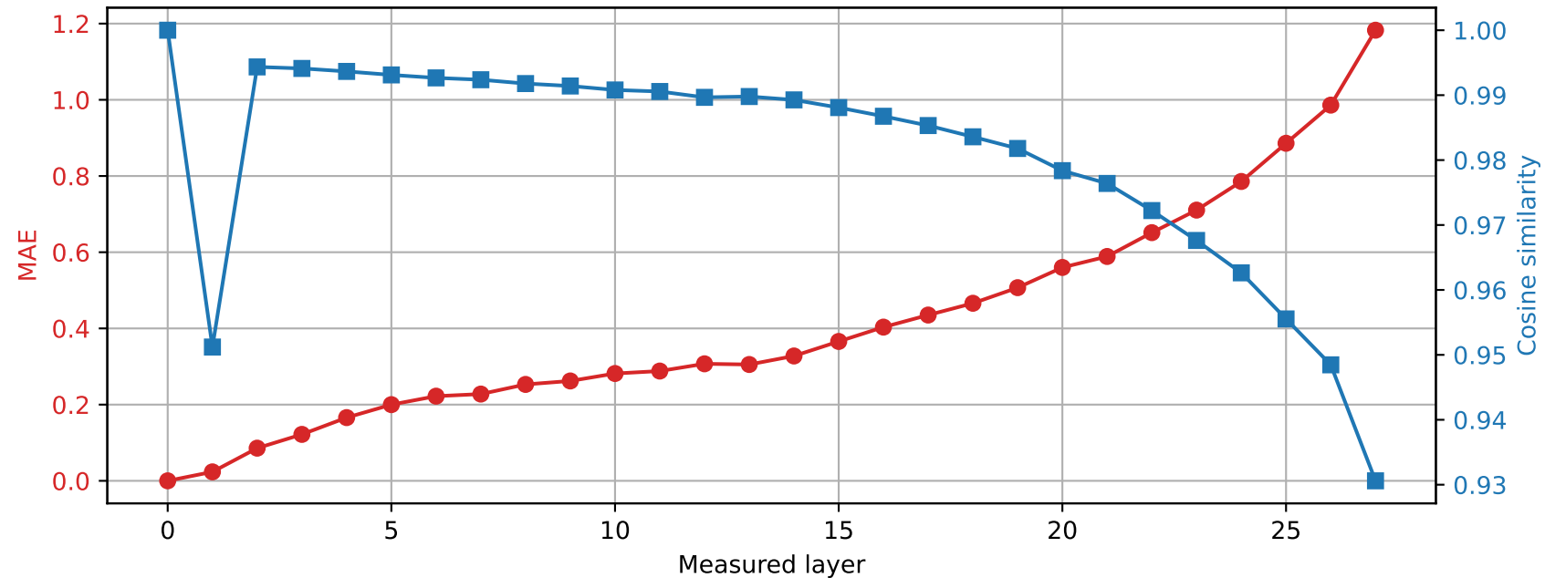
Llama-3.2-3B | Prompt 3 Spared layer 14 | Hybrid vs unquantized
