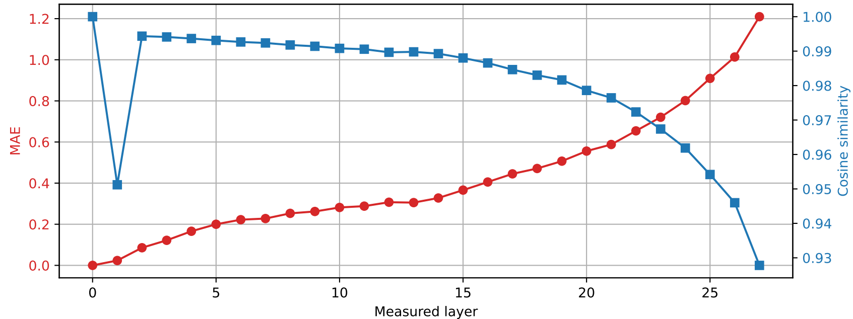
Llama-3.2-3B | Prompt 3 Spared layer 16 | Hybrid vs unquantized
