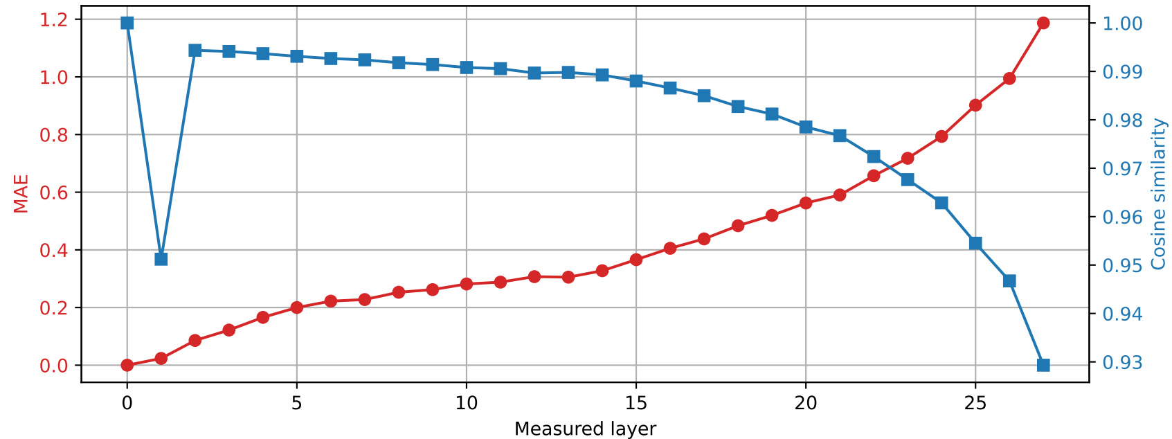
Llama-3.2-3B | Prompt 3 Spared layer 17 | Hybrid vs unquantized
