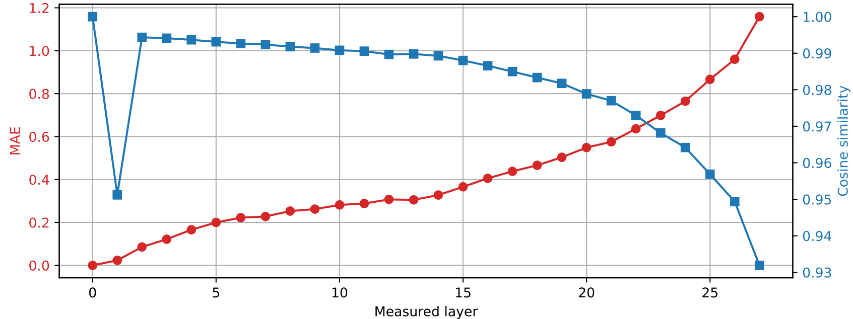
Llama-3.2-3B | Prompt 3 Spared layer 23 | Hybrid vs unquantized
