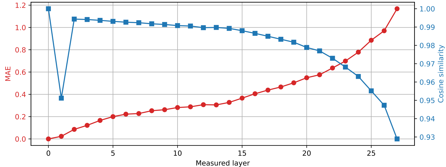
Llama-3.2-3B | Prompt 3 Spared layer 25 | Hybrid vs unquantized
